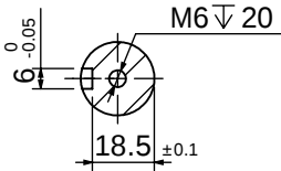
剖面 A-A
