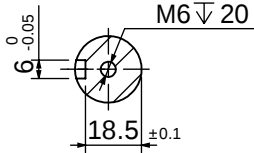
剖面 A-A
