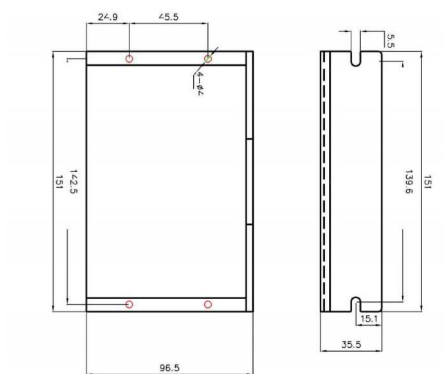
ECR86 安装尺寸
