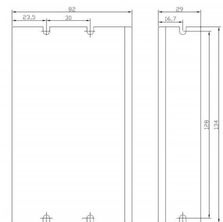
ECR42、ECR60 安装尺寸
