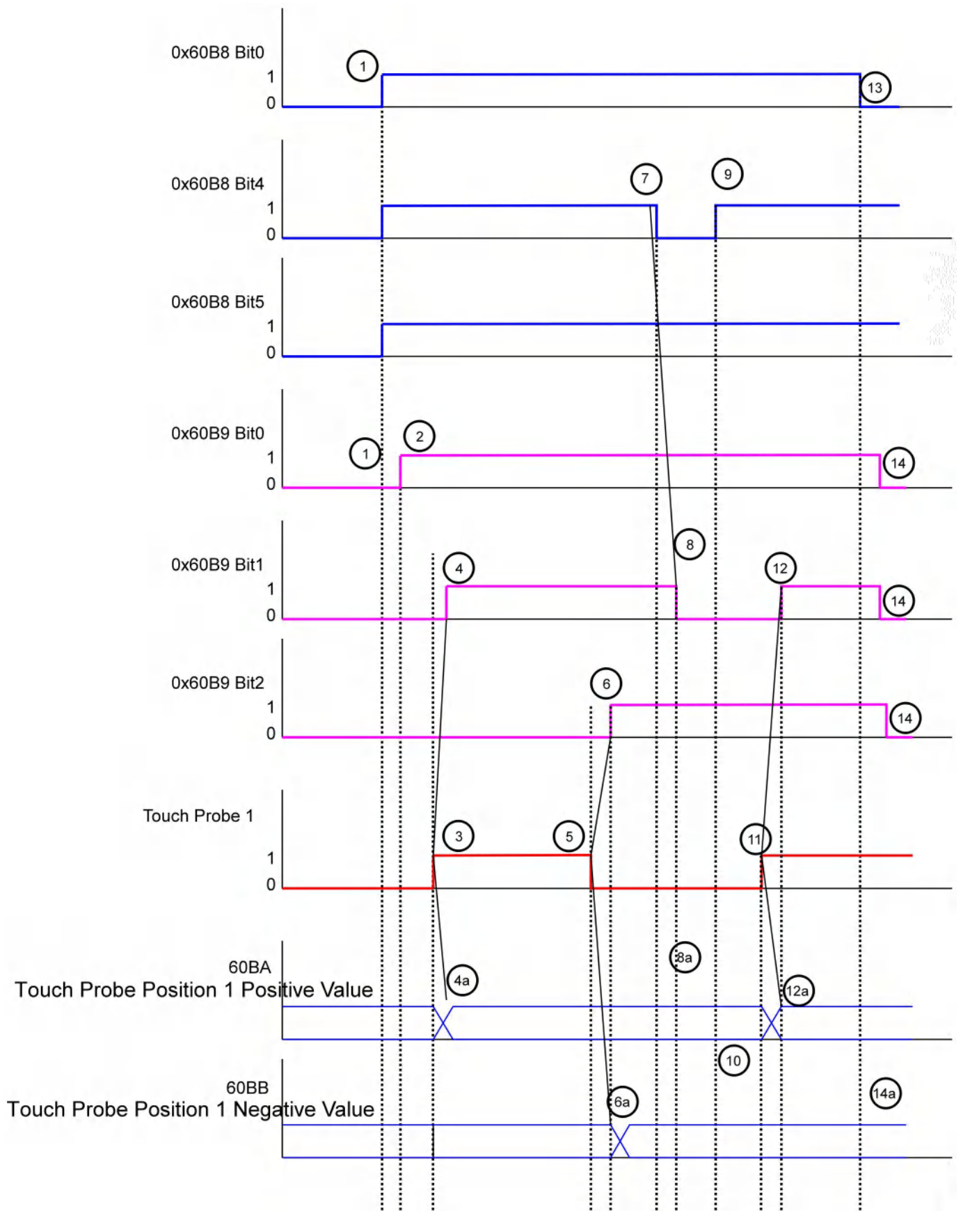
探针时序图
